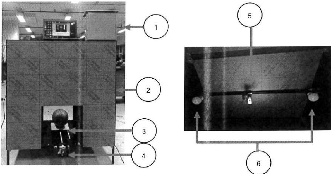
ภาพที่ 6 ส่วนประกอบโครงสร้างเครื่องคัดแยกน้ำหนักเตงโม
