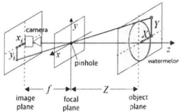
ภาพที่ 5 โมเดลกล้องสำหรับตรวจจับพื้นที่พิกเซล [15]
