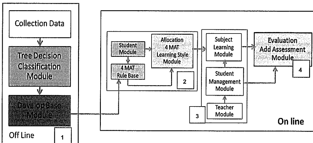
รูปที่ 1 องค์ประกอบของรูปแบบบทเรียนคอมพิวเตอร์ช่วยสอนบนเครือข่ายที่จำแนกผู้เรียนตามความถนัดทางการเรียน ตามทฤษฎี 4 MAT โดยการวิเคราะห์ด้วยวิธีต้นไม้
